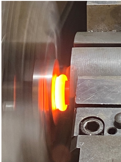
Bild 2: Reibschweißvorgang
